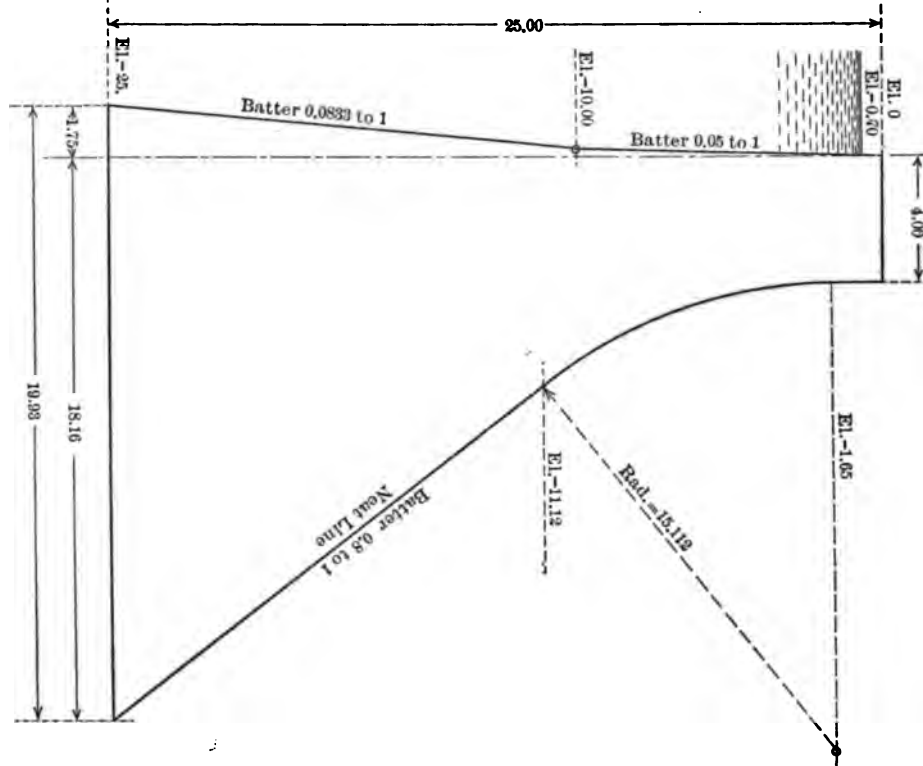
Fig. 1.—TURBINE DAM.
