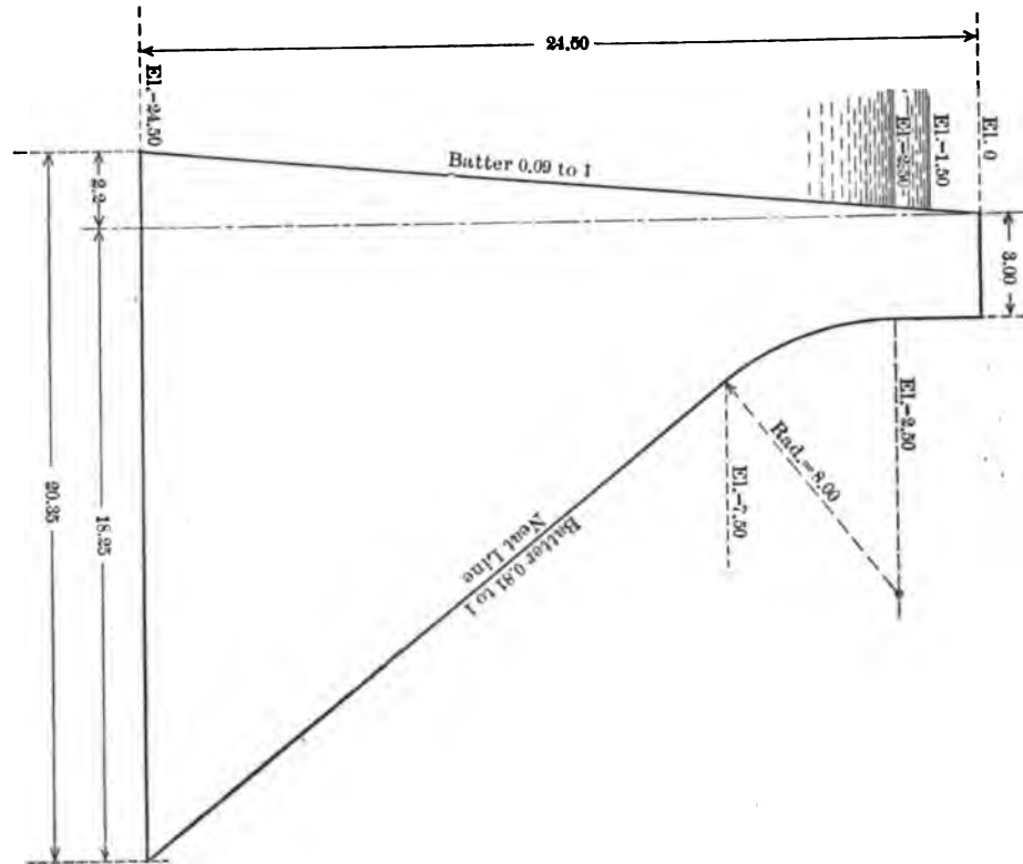
Fig. 2.—MODEREIX DAM.
