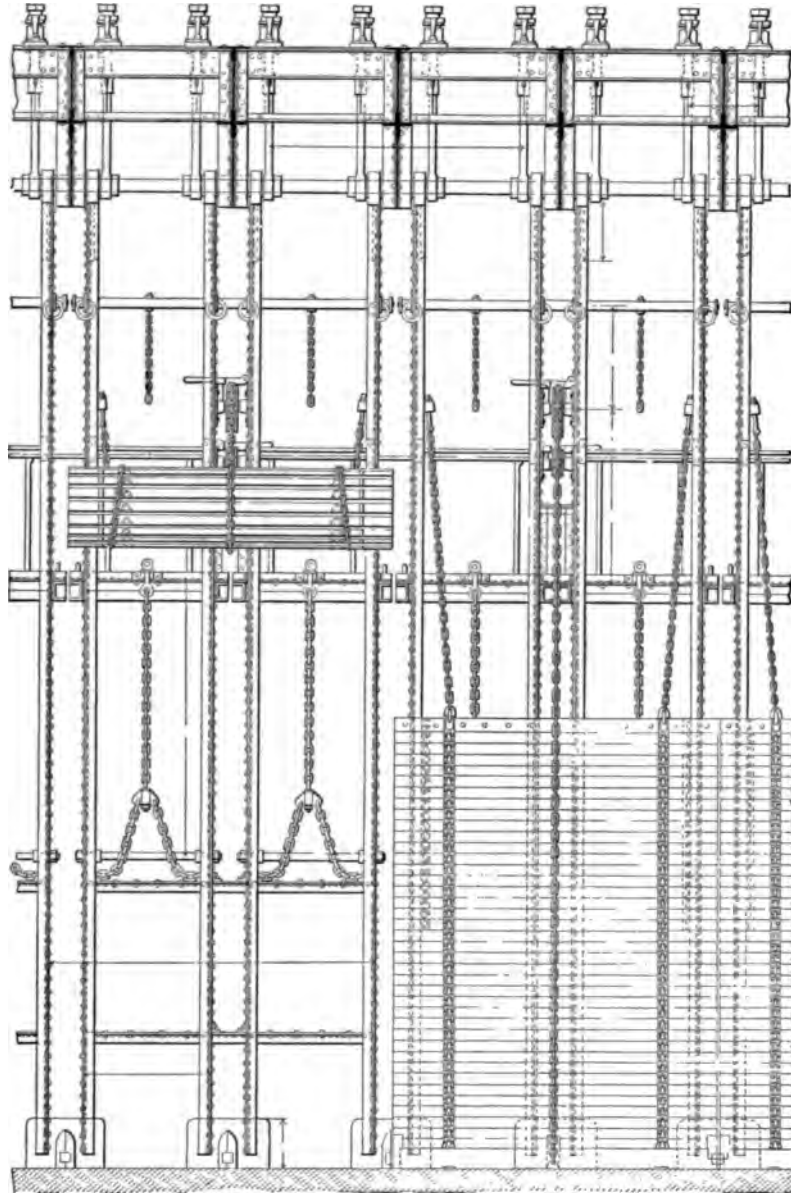
FIG. 84.—CAMÉRE CURTAIN-DAM.
