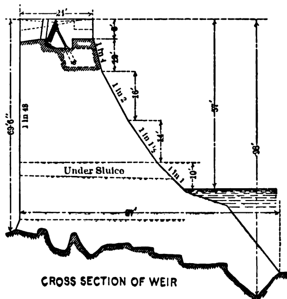
FIG. 34.—FOLSOM DAM.
