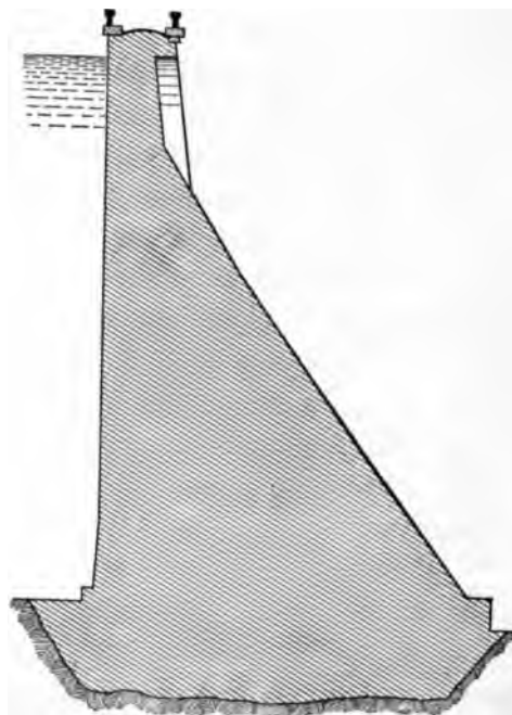
FIG. 28.—THE ECHAPRE DAM.
