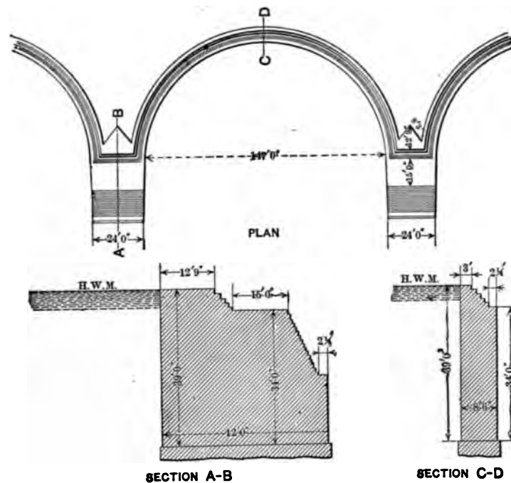
FIG. 31.—MEER ALLUM DAM.
