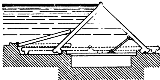
FIG. 110.—CARRO GATE.
