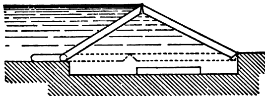
FIG. 109.—DUBOIS GATE.
