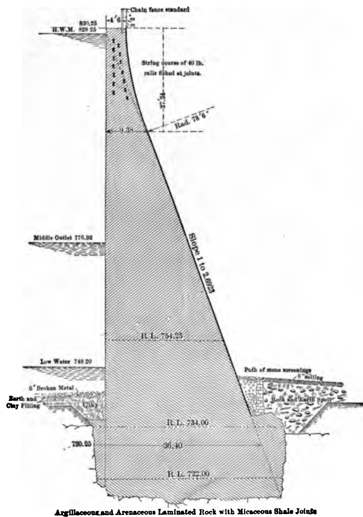
FIG. 32.—BAROSSA DAM.
