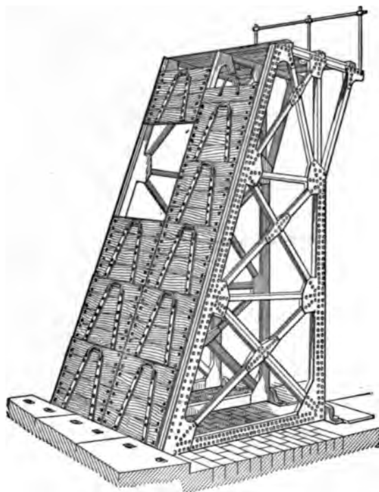
FIG. 82.—BOULÉ GATE.
