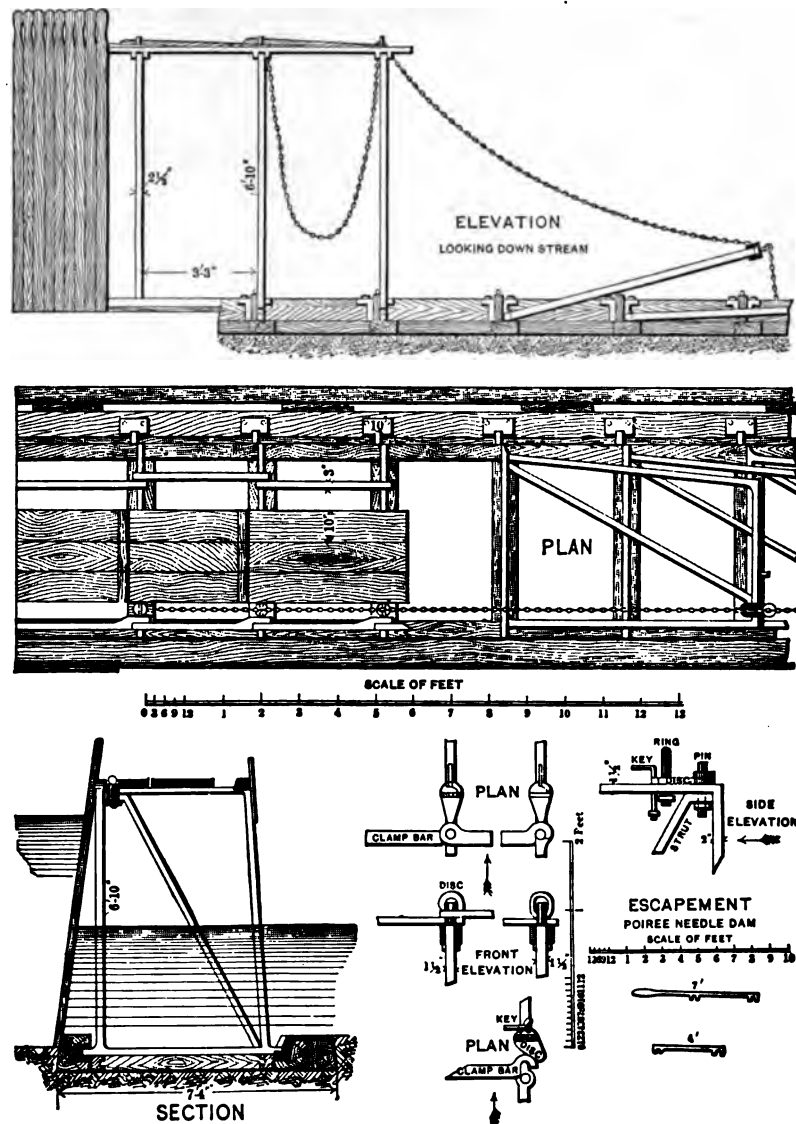
FIG. 77.—POIRÉE DAM.
