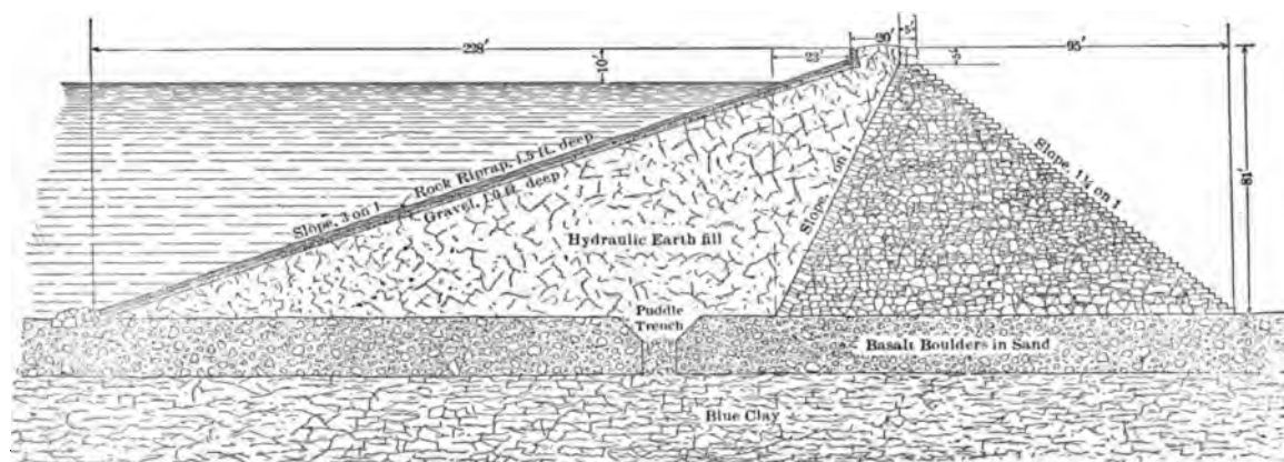
FIG. 58.—ZUNI DAM.
