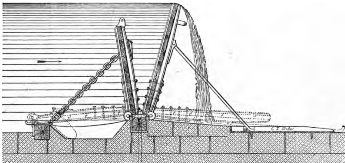
FIG. 93.—THÉNARD SHUTTER-DAM.
